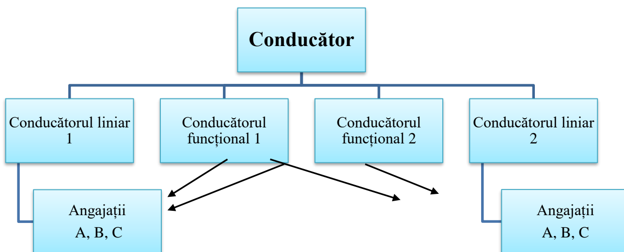
Fig. 3.3. Organigrama liniar-funcțională
